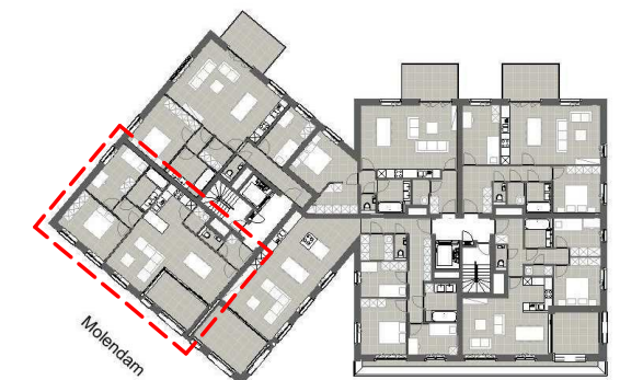
Grondplan
